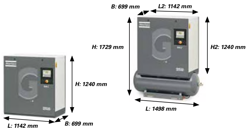
GA 5-7-11 Pack (bodenmontiert)
